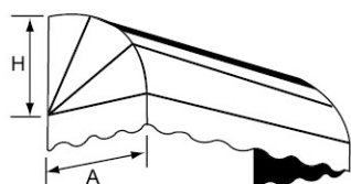
1/ STANDARD - 4 ARCEAUX
